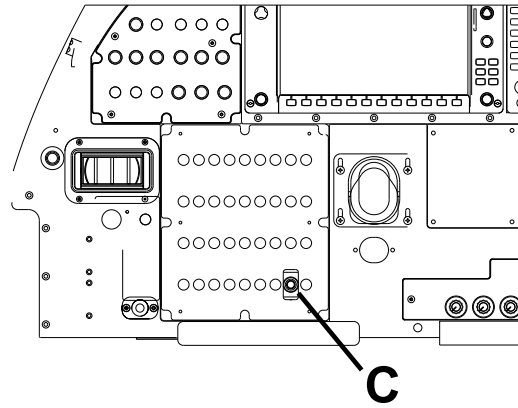
VIEW A-A
